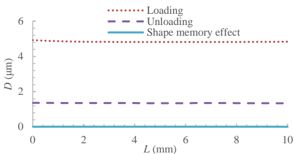
Fig. 10 Crack opening distance at the end of each step for two wires شکل 10 بازشدگی ترک در انتهای هر مرحله برای دو سیم
