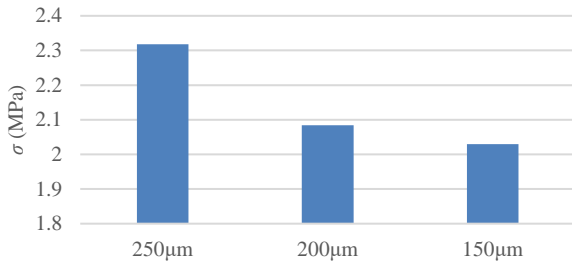
Fig. 12 Ultimate fracture stress in the model with different wire radius شکل 12 تنش نهایی شکست در نمونه با سیم‌های با شعاع متفاوت
